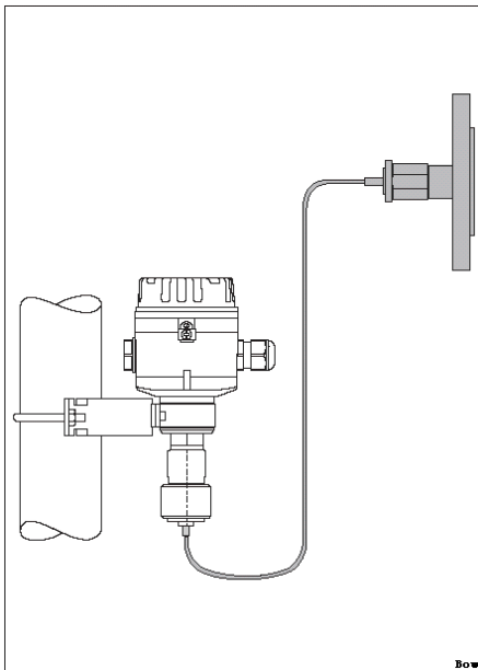
毛细管安装 (max. +350℃)
